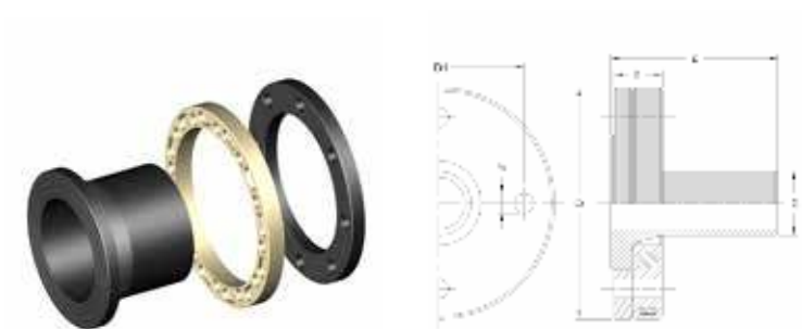
Тип В - втулка под фланец, стальной фланец и ПП кольцо
