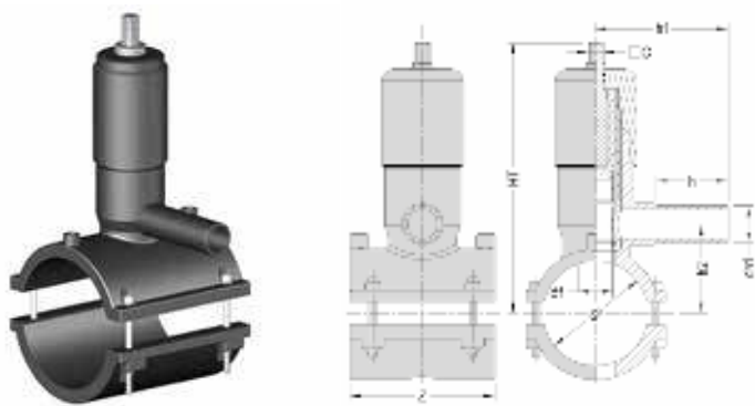
□C = штанга управления с квадратным клиновидным креплением
